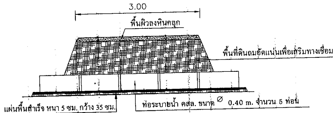
แบบแสดงรูปตัดการฝังท่อและทำทางเชื่อม จุดที่ 2
